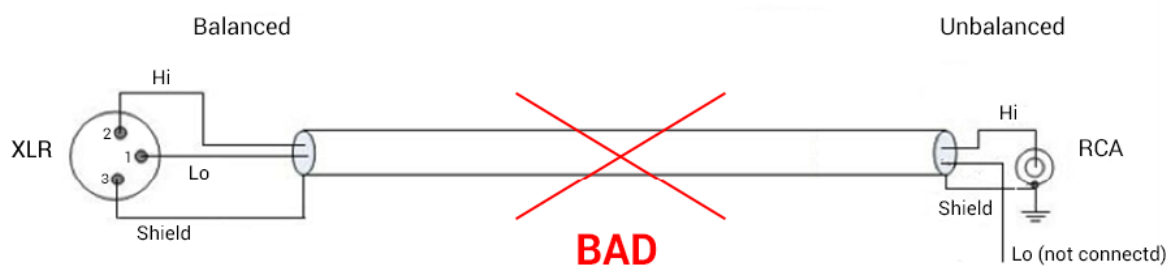
Figure 3 Anubis出力をアンバランス入力に接続する間違った方法
